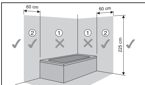
Fig. 18 Zona de protección
