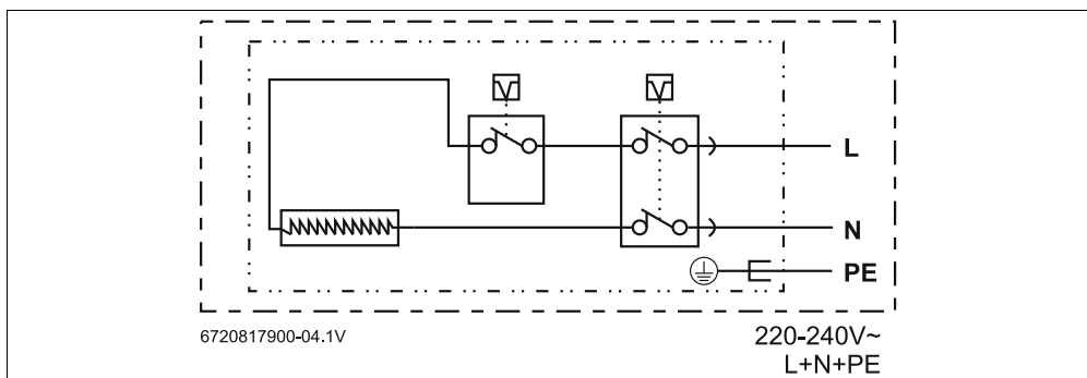
Fig. 24 Esquema de conexiones
