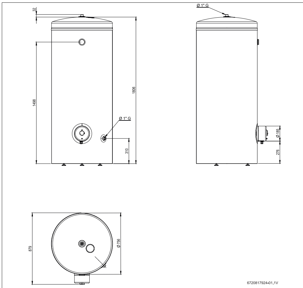
Fig. 14 Dimensiones en mm
