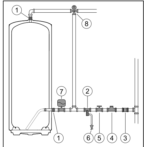
Fig. 20 Toma de agua
