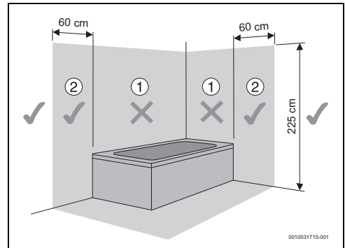
Fig. 6 Área de proteção
