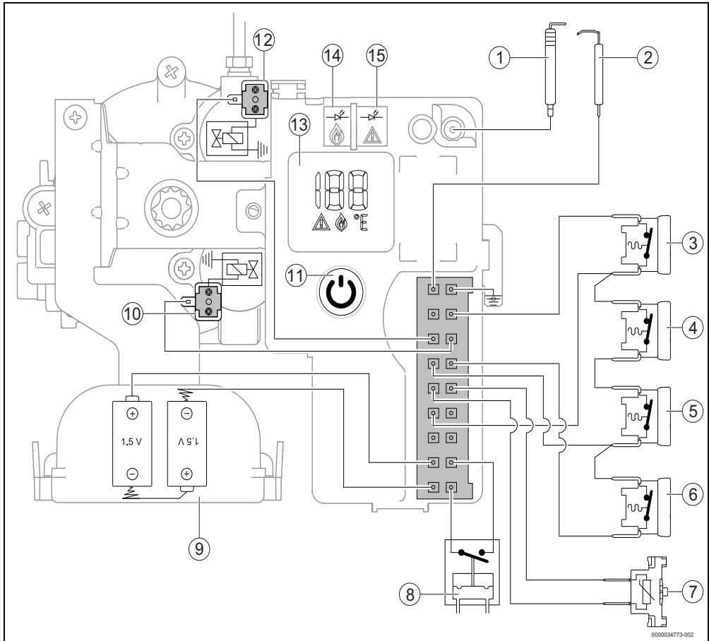
Fig. 30 Esquema elétrico
