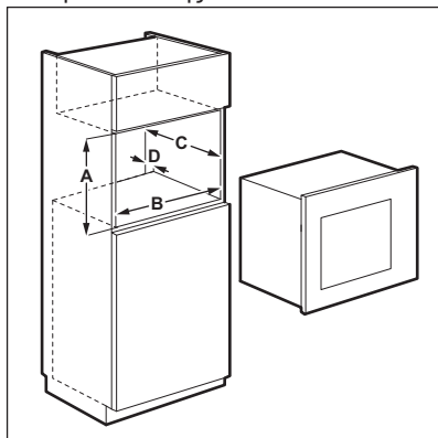
Αποστάσεις εγκατάστασης
