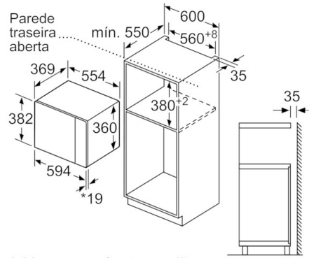
* 20 mm para frente metálica Medidas em mm
